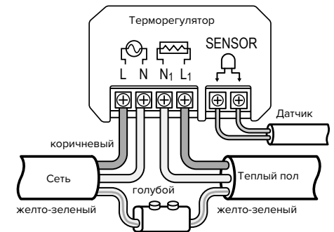
Подключение к 2-х проводной линии
