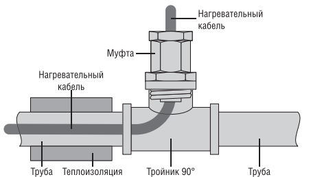
Схема 4. Монтаж муфты в тройник 90°
