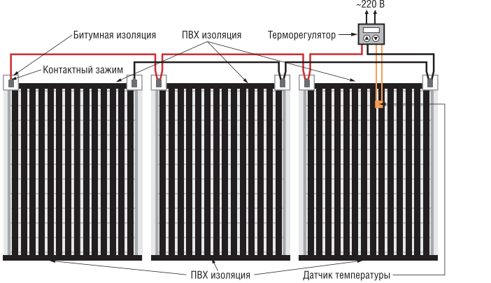
Рис. Общая схема подключения термоплёнки CALEO PLATINUM
