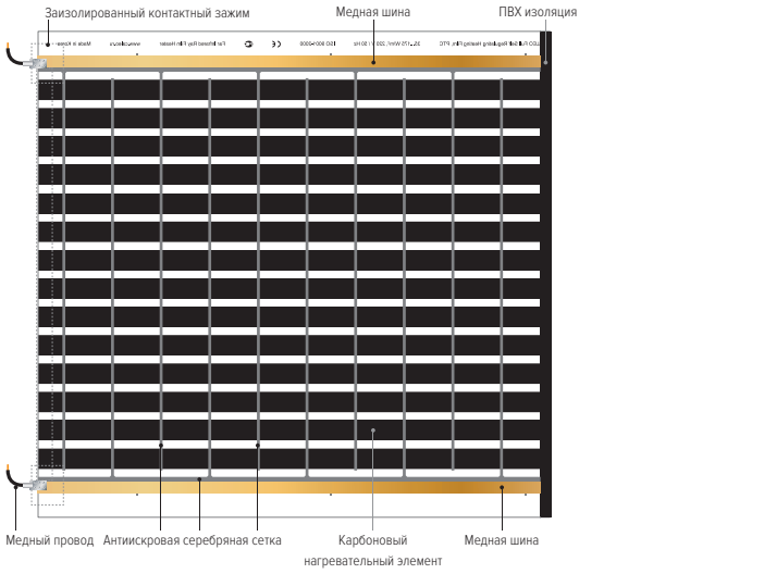
Рис. Общий вид термоплёнки CALEO, расположение основных ее элементов, контактных зажимов и мест подключения и изоляции
