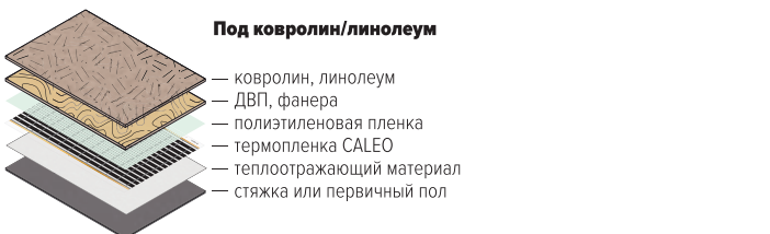
Рис. Схема монтажа теплого пола CALEO под ламинат, ковролин, линолеум
