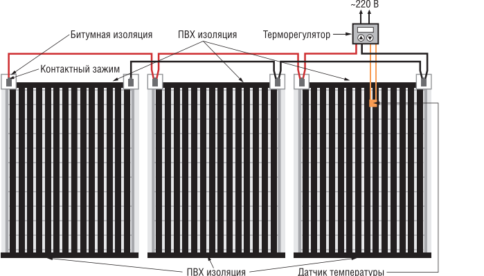
Рис. Общая схема подключения термопленки CALEO PLATINUM
