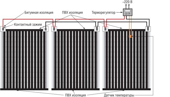
■ Заизолированный контактный зажим
