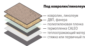
Рис. Схема монтажа теплого пола CALEO под ковролин или линолеум
